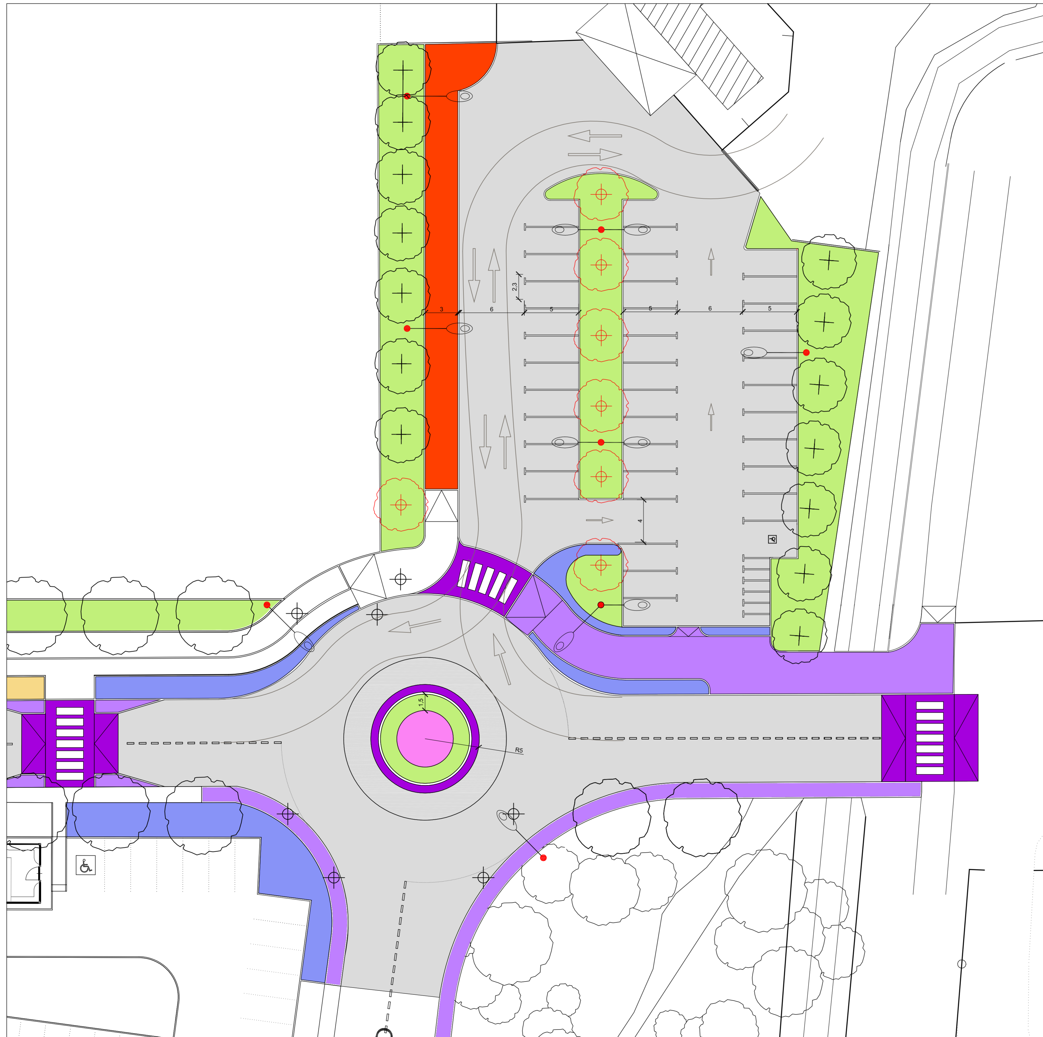
1 Planimetria scala 1:200
